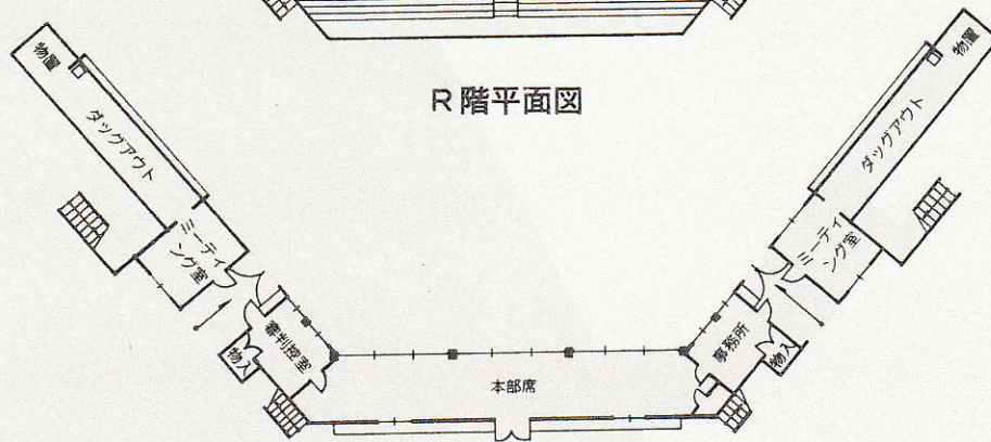
1 階平面図
